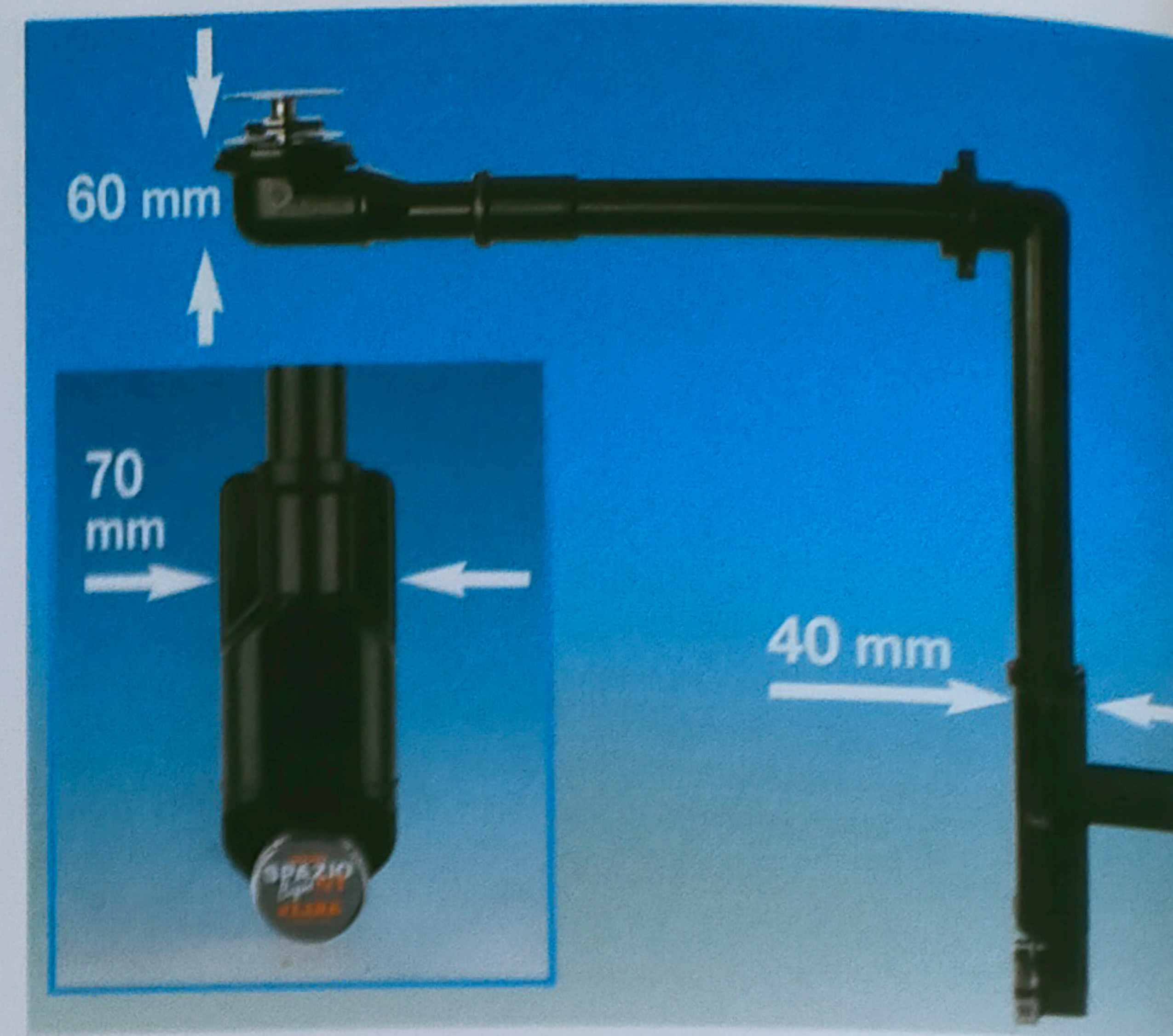
PLATZBEDARF DES SIPHONS
